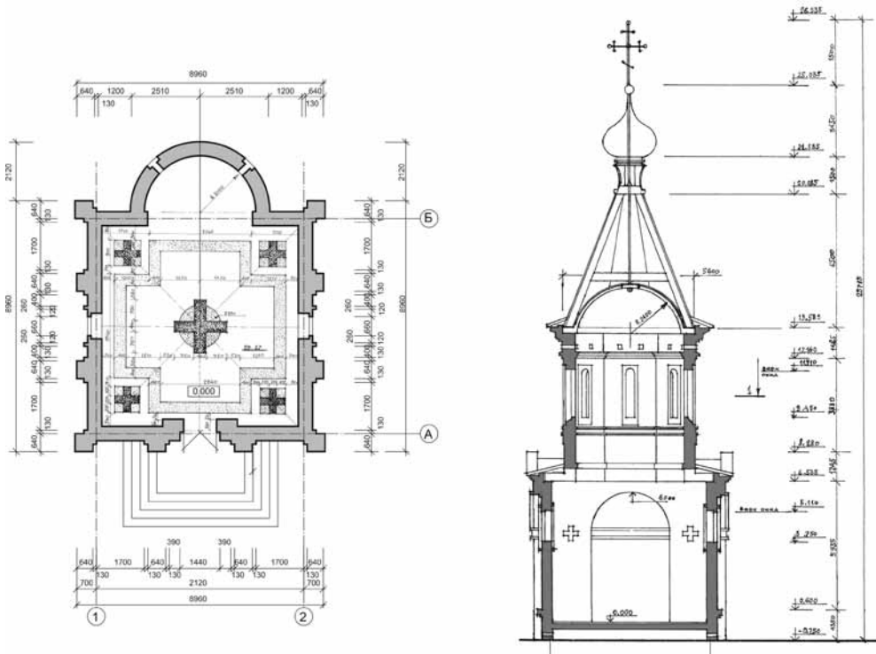
Чертеж храма-часовни св. мч. Виктора
