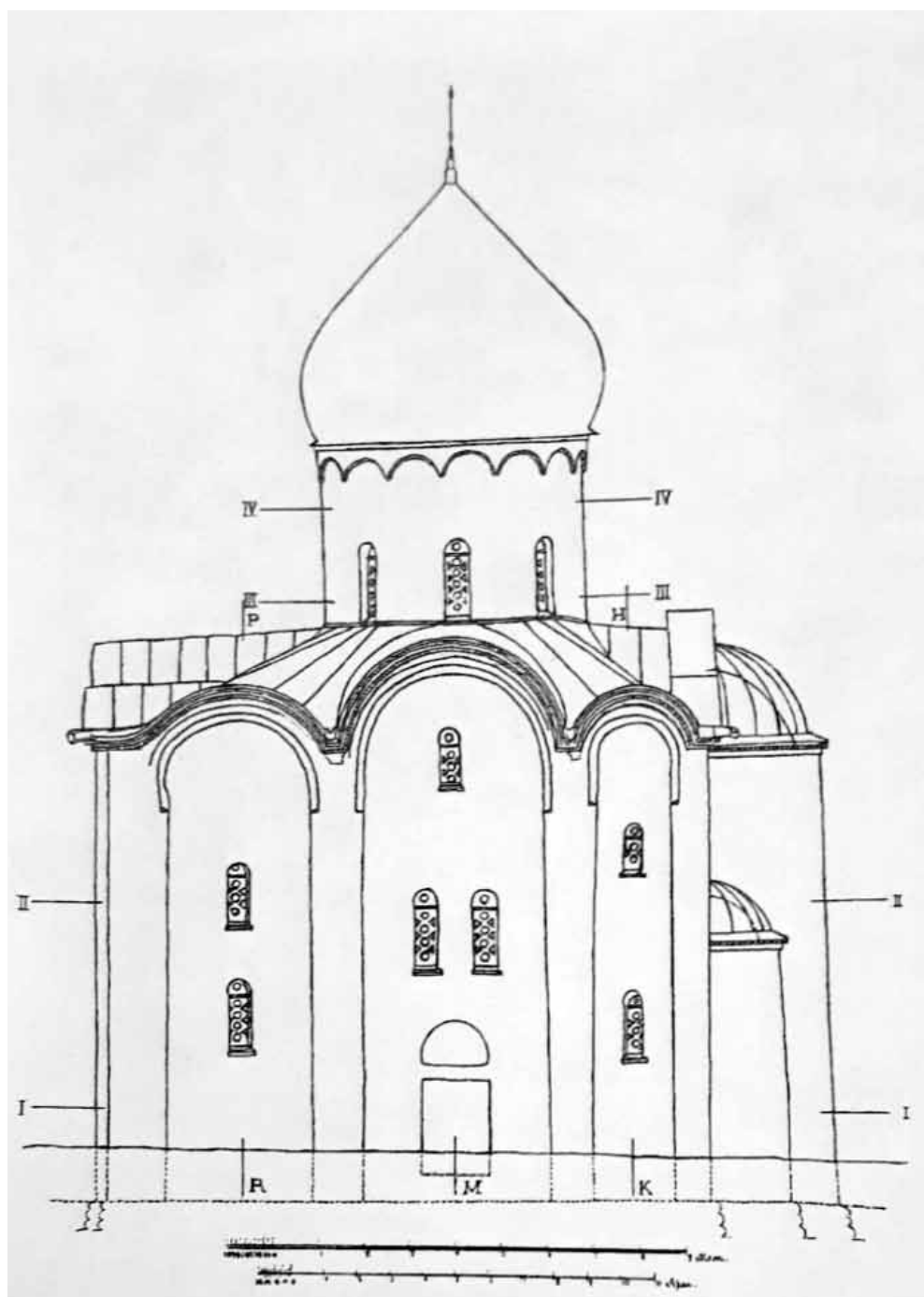
Ил. 6. Церковь Спаса Нередицы. Южный фасад. Проект реставрации П. Покрышкина. 1903 г. ИИМК РАН
